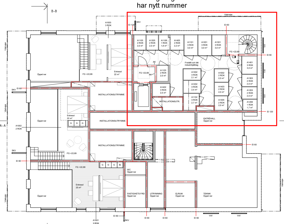
Plan 10 Entresol
