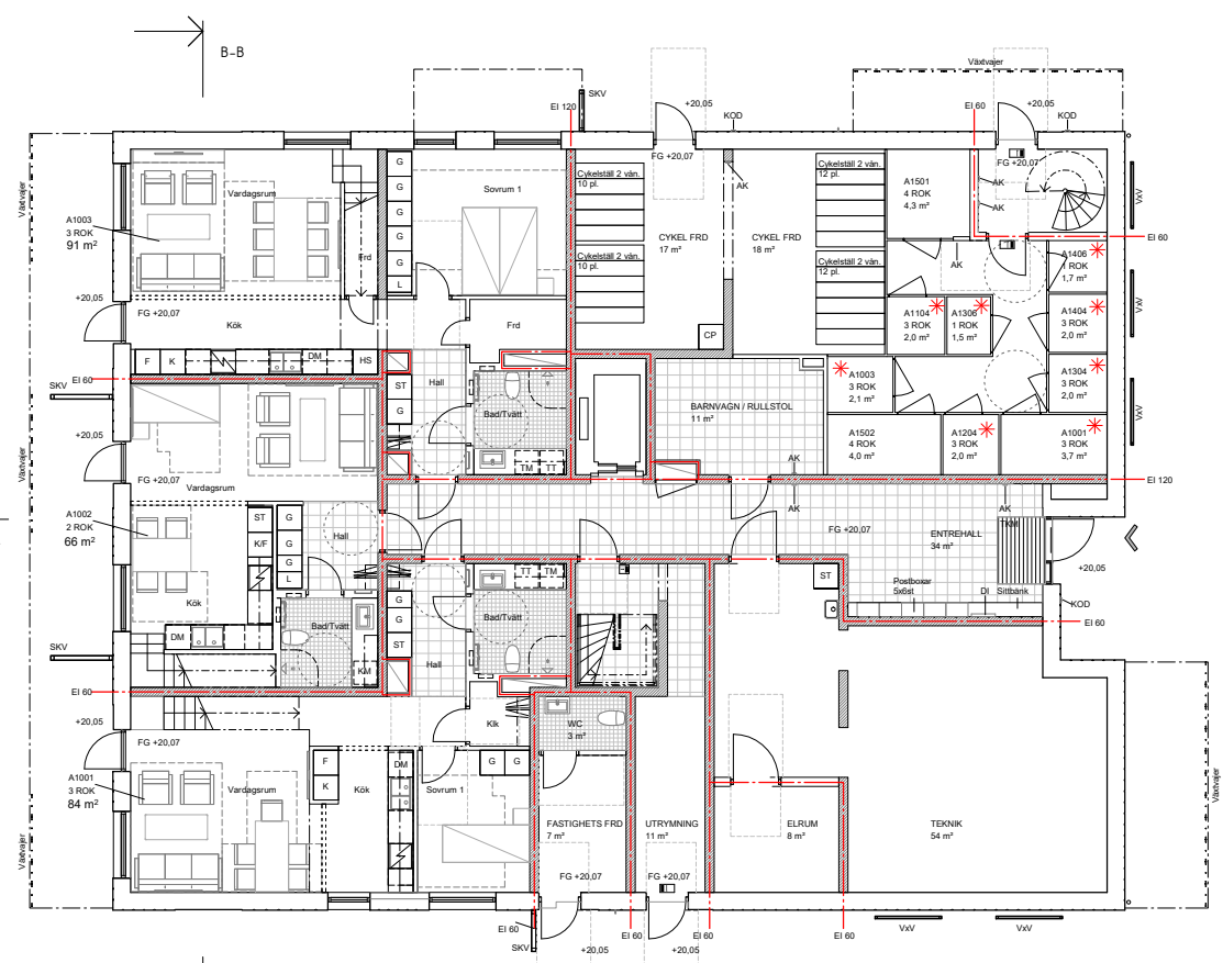
Plan 10 Entréplan
