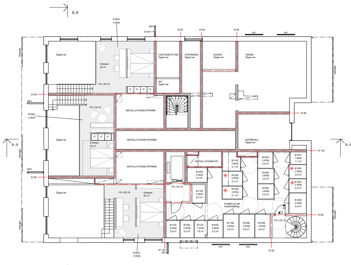
Plan 10 Entresol
