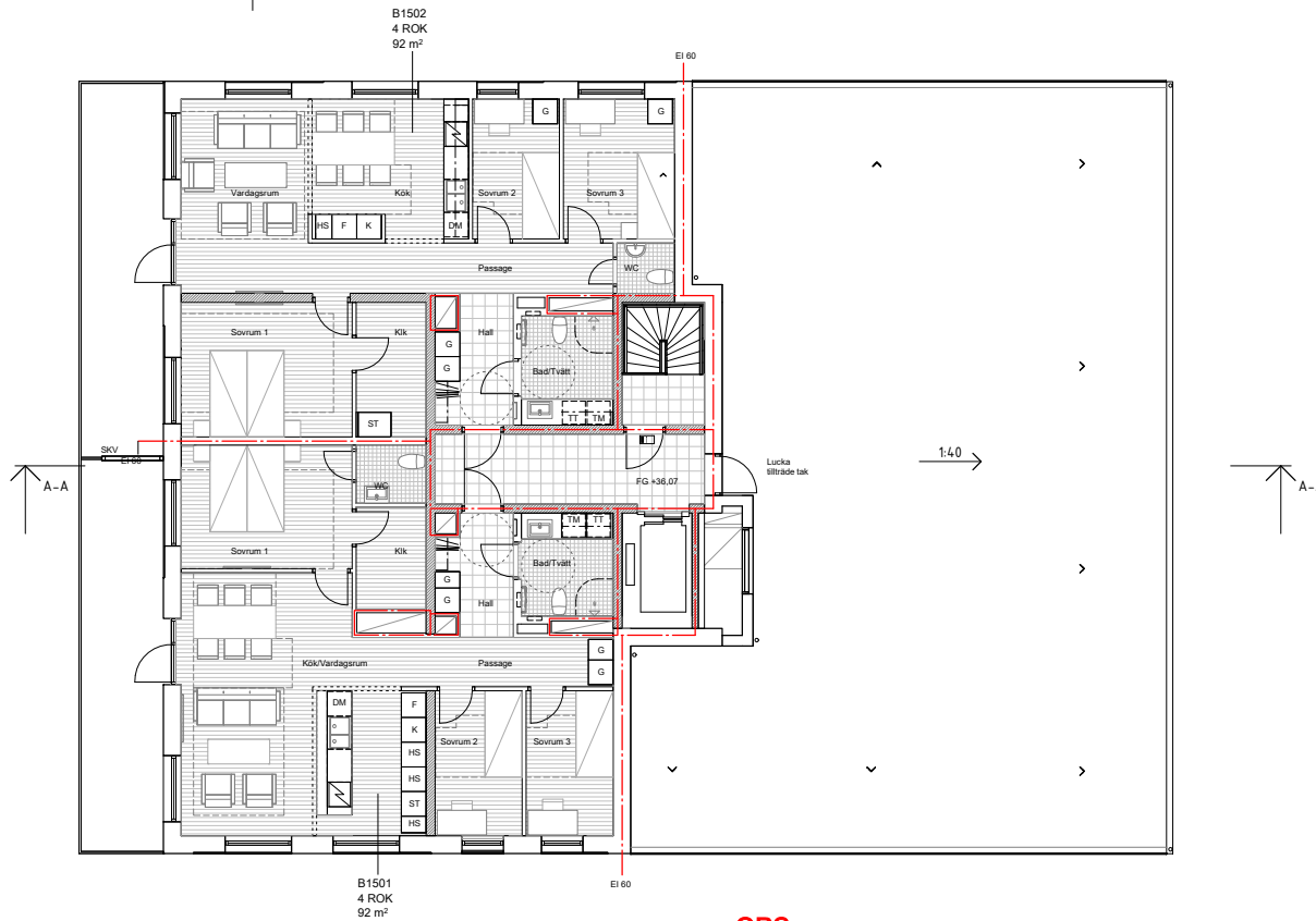
Plan 15 Takväning
