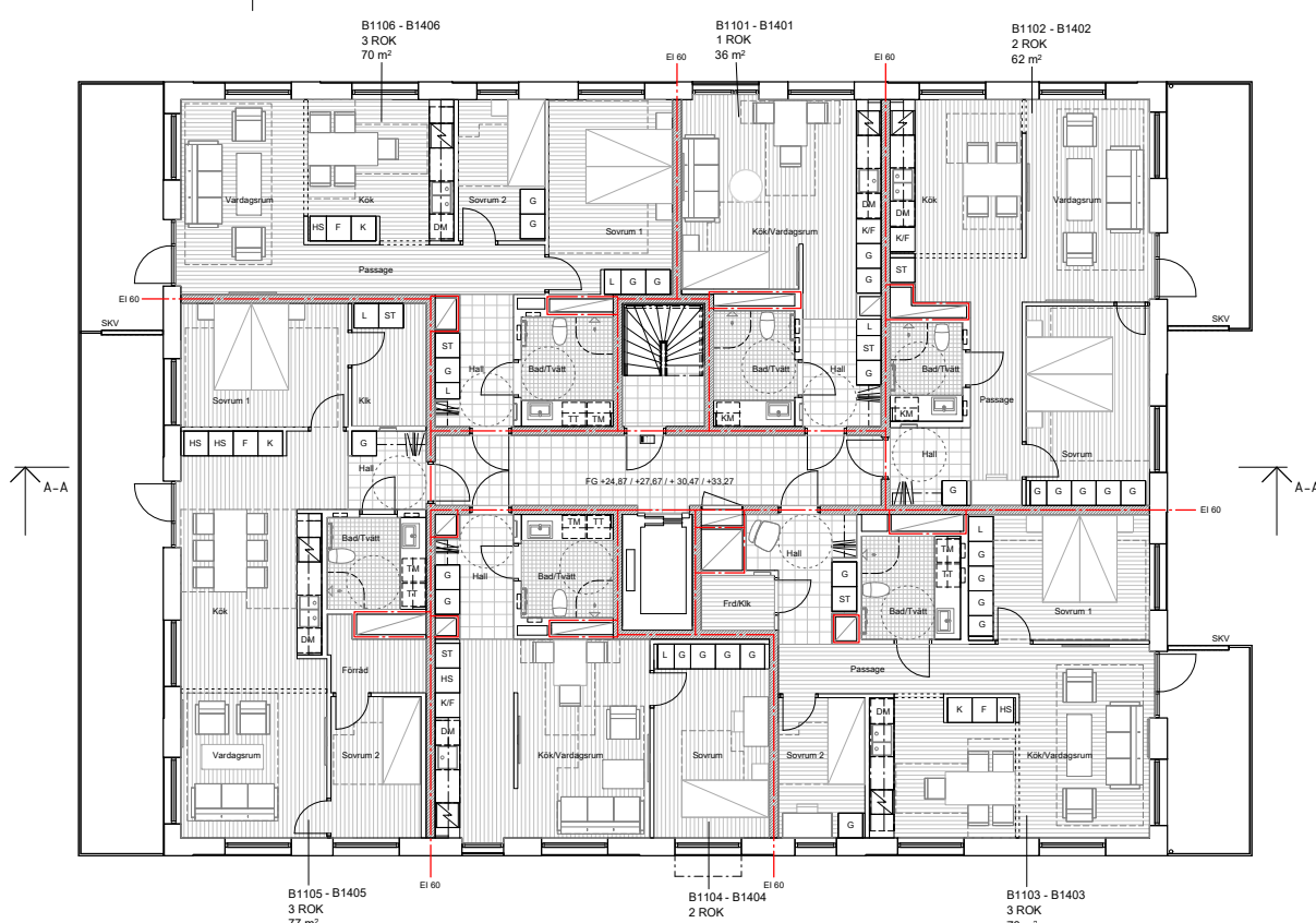
Plan 11-14 Normalplan
