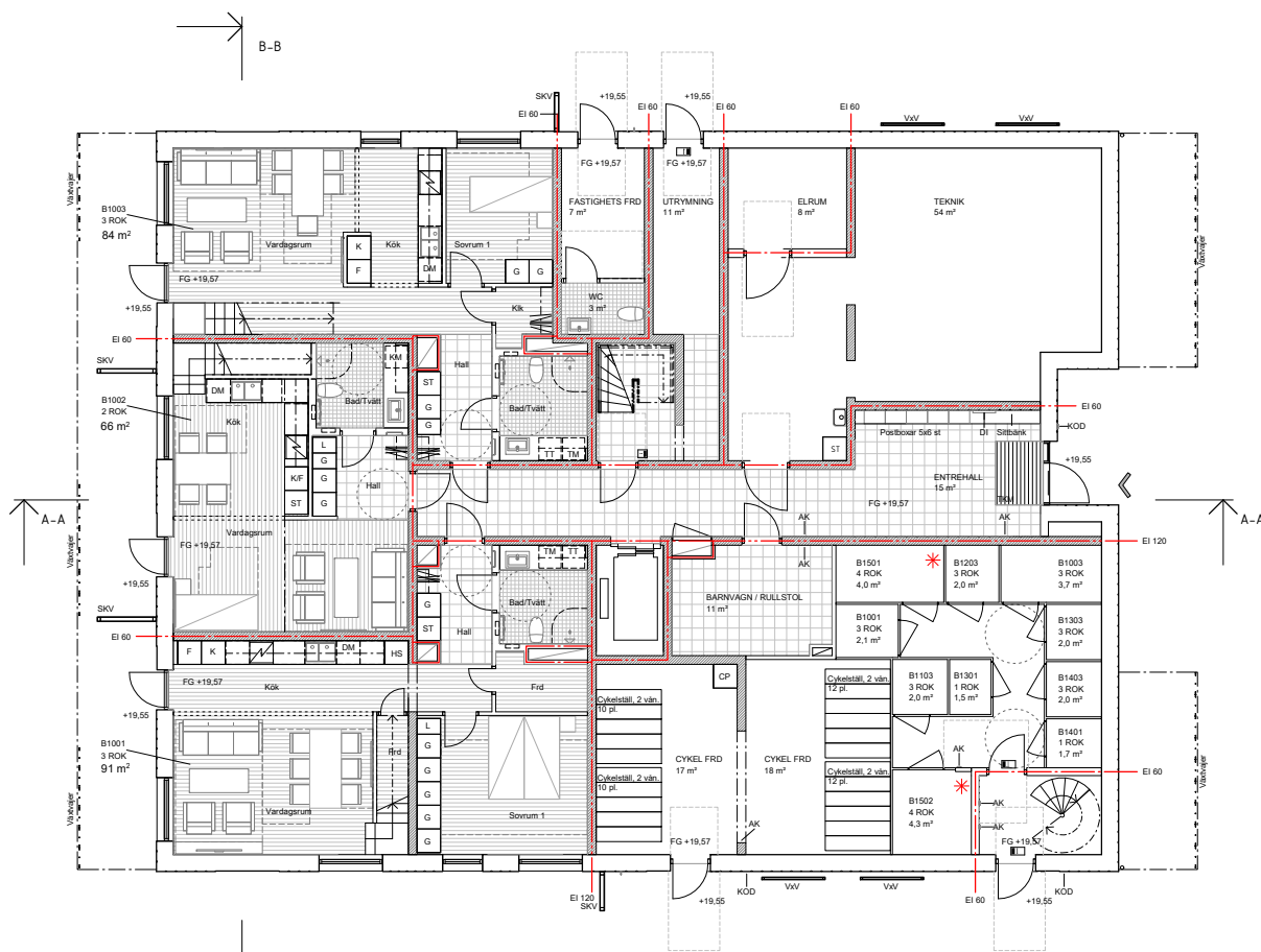
Plan 10 Entréplan
