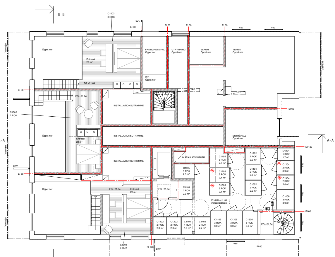
Plan 10 Entresol
