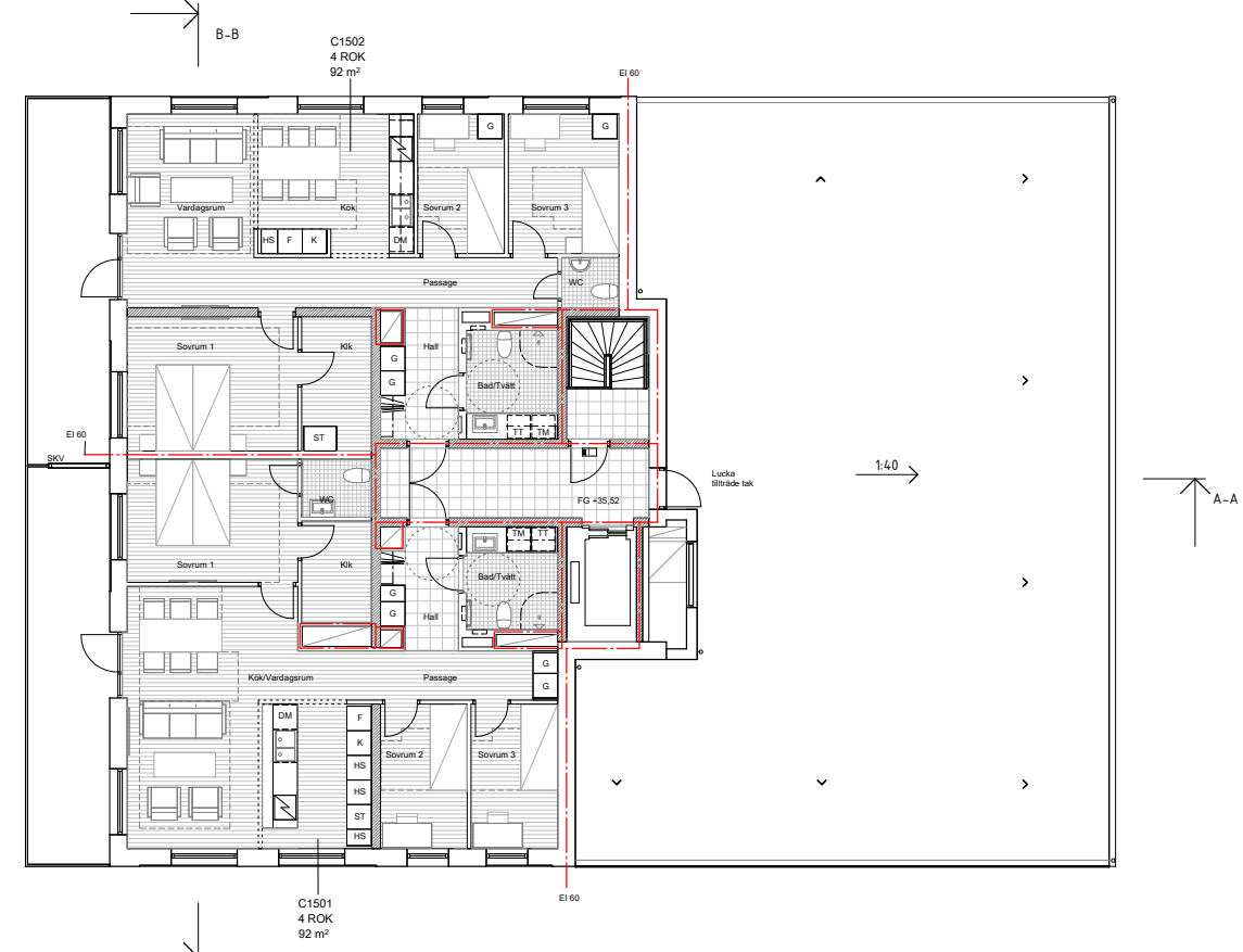
Plan 15 Takvåning
