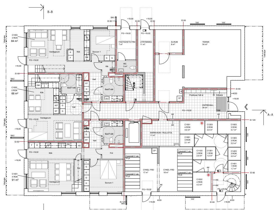
Plan 10 Entréplan
