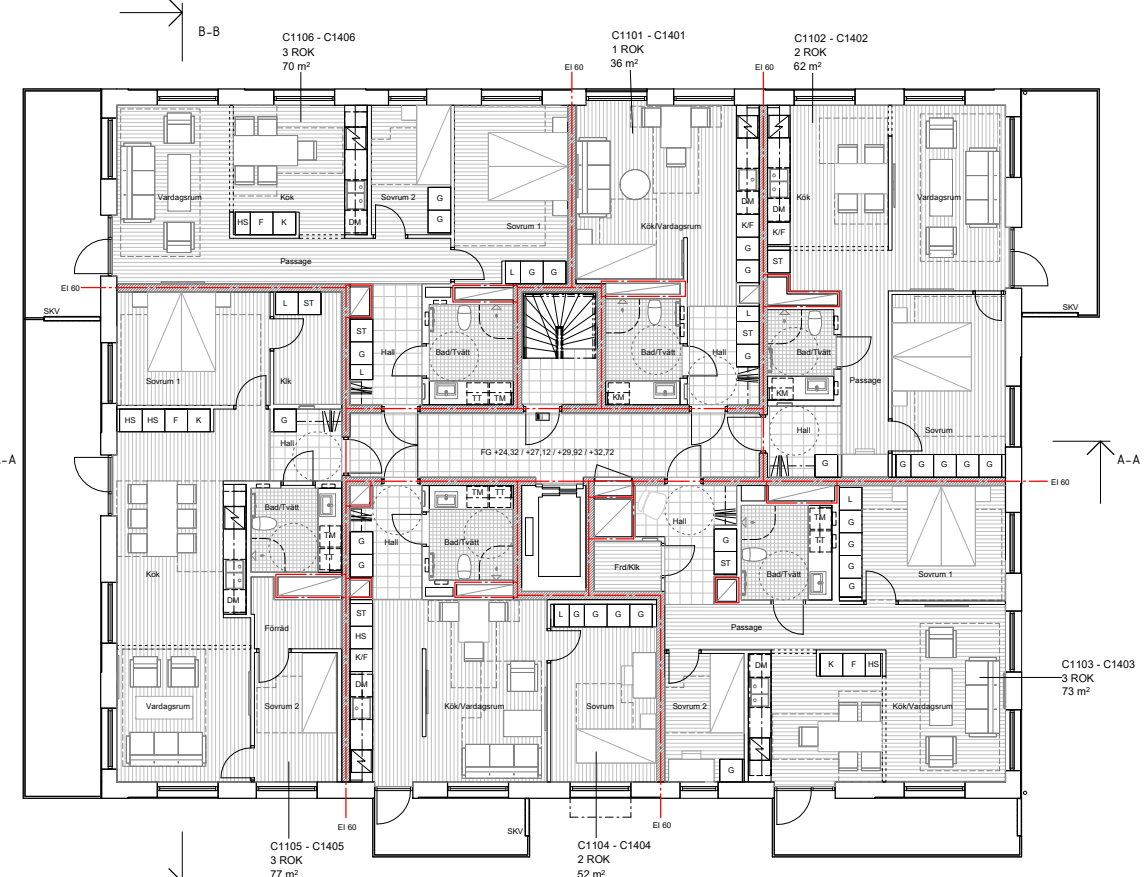
Plan 11-14 Normalplan
