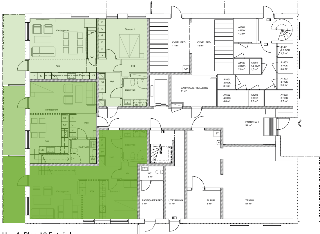
Hus A, Plan 10 Entréplan
